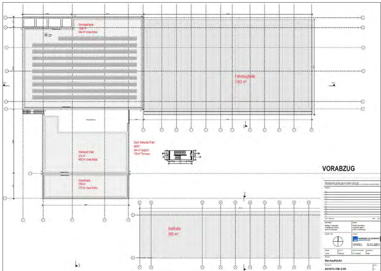
Abbildung 2: Auszug der Dachaufsicht der geplanten Gebäude (Stand: 31.10.2024). Quelle: Arc-Architekten.
